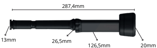
3265 - Insuflador IP13U-MV - Teteira triangular
