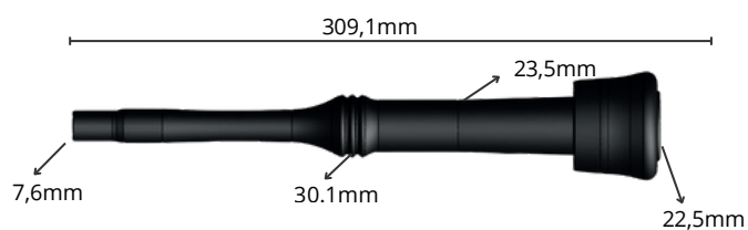
1264 - Insuflador WF 030 U XP
