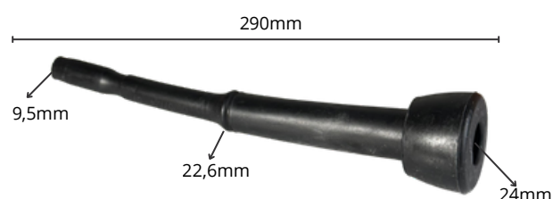
1451 - Teteira 1 anel 9,5mm S/Marca S
