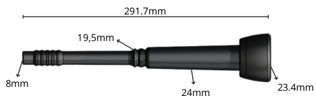
1271 - Insuflador AL 1U XP
