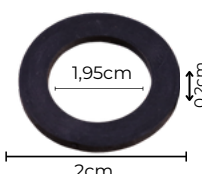
2542 - Anel vedação abraçadeira
