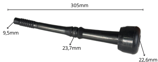
6467 - Teteira borracha Mod. WF Fast Flow cor preto
