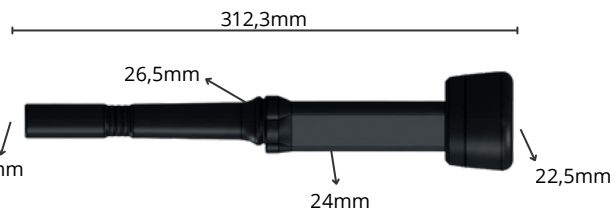
7505 - Insuflador IP10U ( não ventilada )
