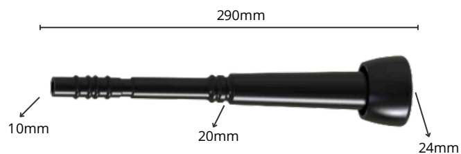
6645 - Teteira Mod. 2 anel inter SM 10mm
